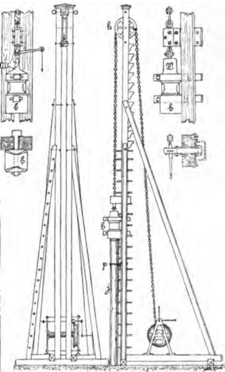
Č. 531. Beranidlo strojové.
